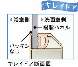
クレイドア断面図
